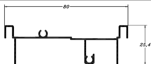
PBA 0471 (IBL4044-BEL044) TRILHO 2 FOLHAS E 4 FOLHAS SUPERIOR 0,494 Kg/m
