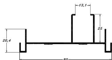
PBA 1120 (IBL4052-BEL052) LATERAL 2 FOLHAS E 4 FOLHAS COM FOLHAS 0,468 Kg/m
