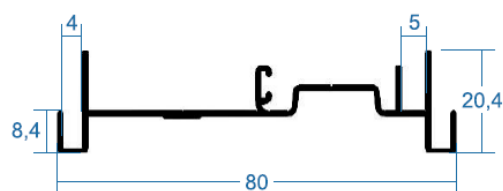
PBA 1132 (IBL4037-BEL037) LATERAL 2 FOLHAS COM ACABAMENTO 0,451 Kg/m
