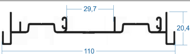
PBA 0474 (IBL4045-BEL045) TRILHO 3 FOLHAS E 6 FOLHAS SUPERIOR 0,636 Kg/m
