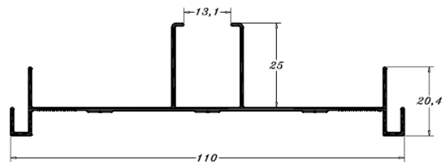
PBA 1121 (IBL4053-BEL053) LATERAL 3 FOLHAS 6 FOLHAS COM FOLHAS 0,550 Kg/m
