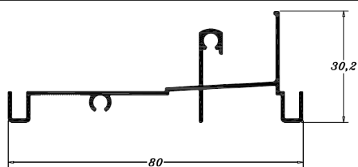
PBA 0467 (IBL4043-BEL043) TRILHO 2 FOLHAS E 4 FOLHAS INFERIOR 0,489 Kg/m
