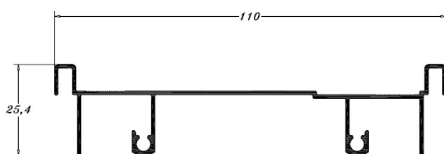
PBA 0474 (IBL4045-BEL045) TRILHO 3 FOLHAS E 6 FOLHAS SUPERIOR 0,636 Kg/m
