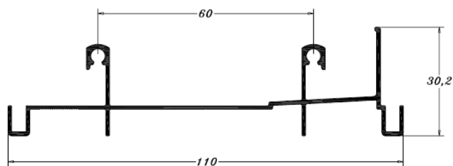
PBA 0473 (IBL4046-BEL046) TRILHO 3 FOLHAS E 6 FOLHAS INFERIOR 0,653 Kg/m
